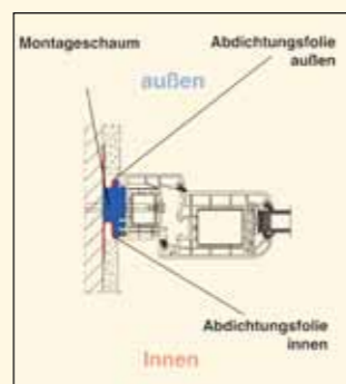
Dichtband
