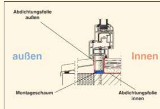
Anschluss Aluminium-Fensterbank
