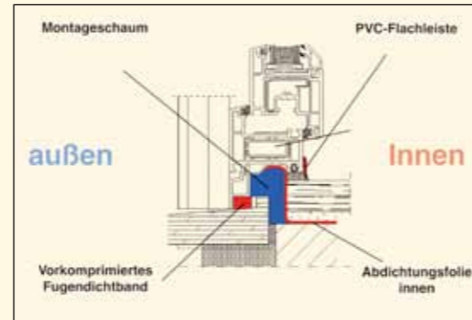
Anschluss Stein-Fensterbank
