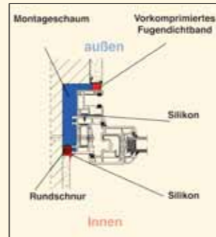
Anschlag mit Rolladenführung
